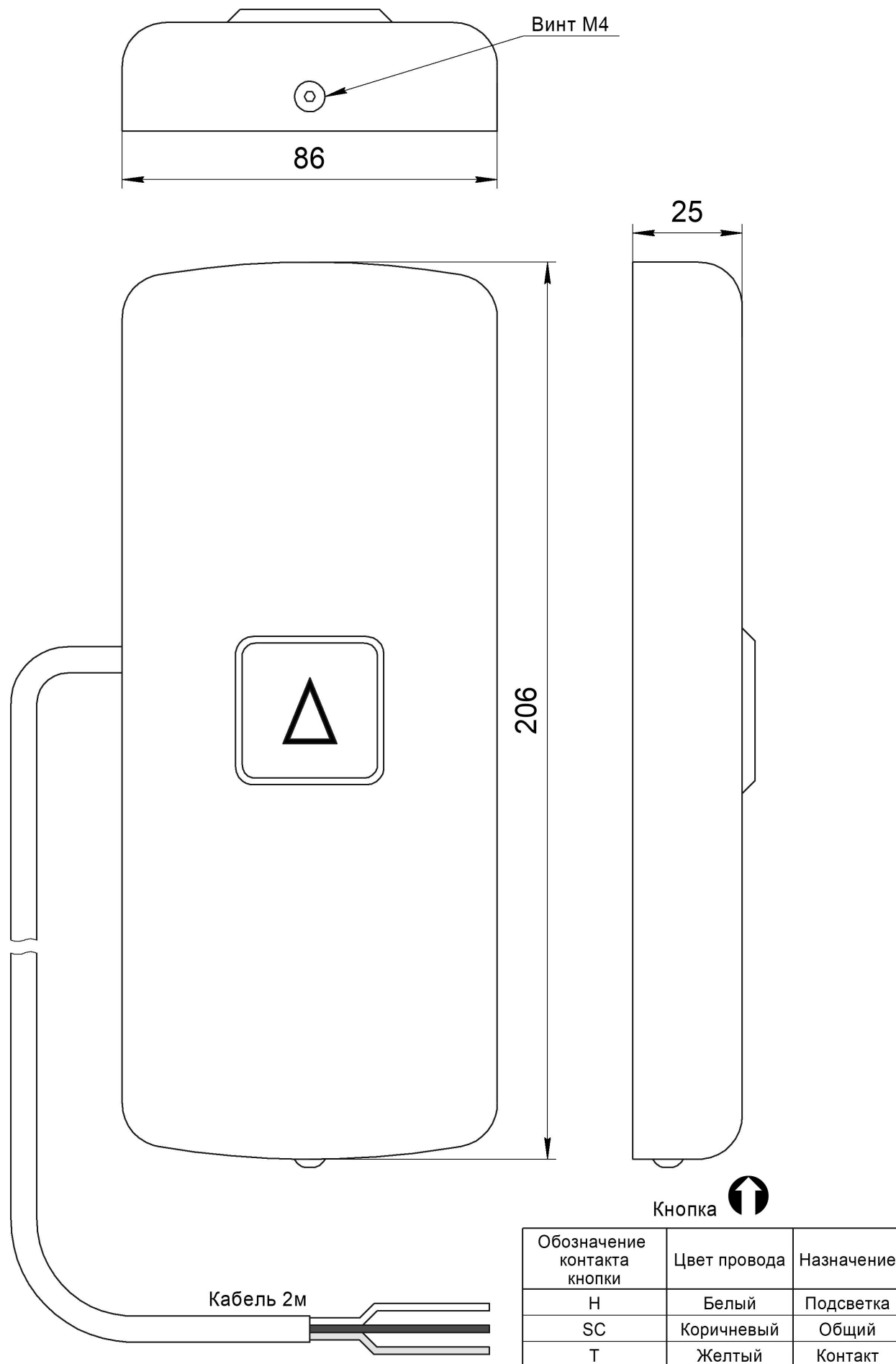
Рис.1 Внешний вид и габаритные размеры Вызывного поста ВП-1001-01
